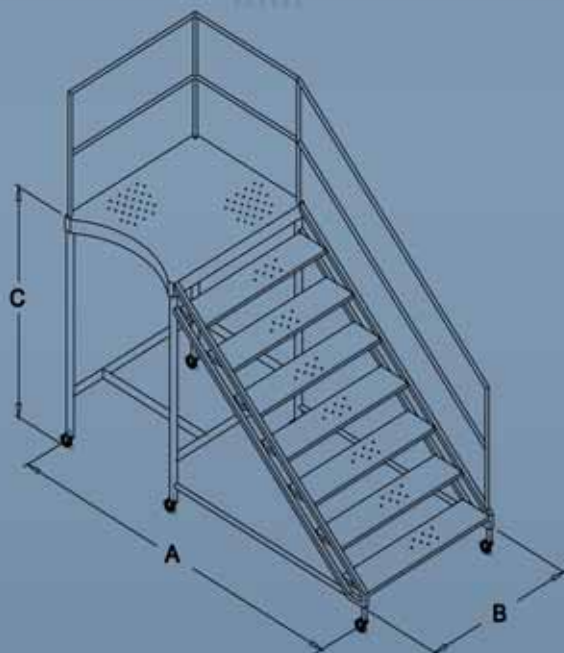
VISTA ISOMÉTRICO
