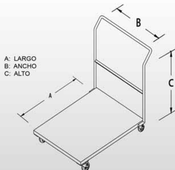
VISTA ISOMÉTRICO
